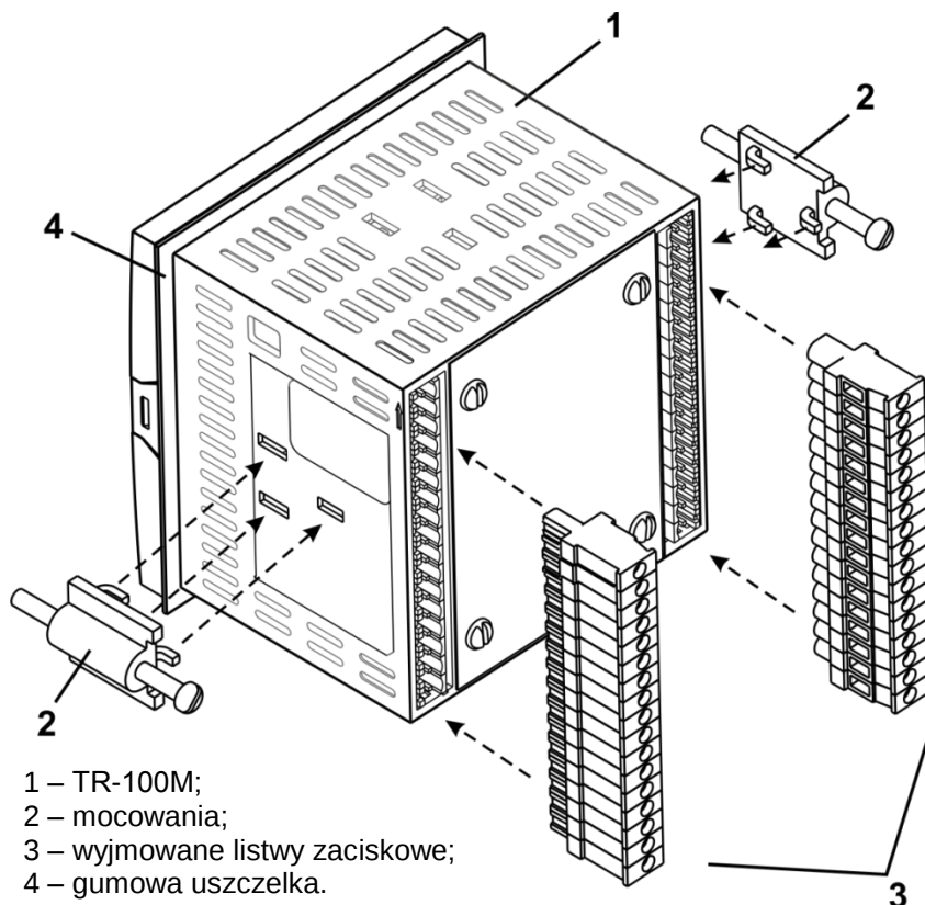
Rysunek 5.1- Montaż urządzenia
