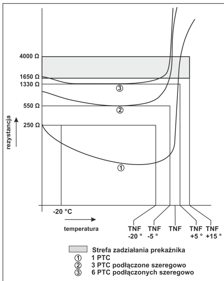
Rysunek 5.3. Wykres zależności rezystancji czujnika PTC od temperatury
